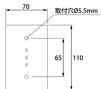
ベースパッキン寸法図
